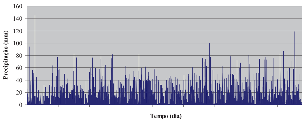
Figura 3: exemplo de série histórica de chuvas diárias de um posto pluviométrico (BRASIL, 2001b)
